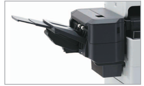
Optionaler Multi-Finisher mit einer Ausgabekapazität von 500 Blatt und einer Heftkapazität bis zu 50 Blatt
